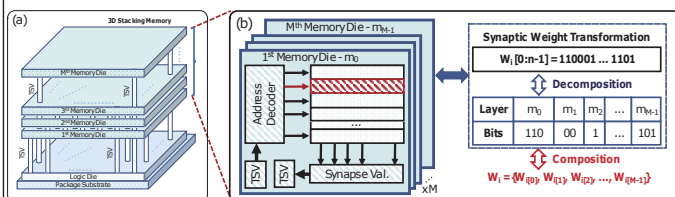
3D-ICベースのニューラルネットワークシステムの概要： (a) 多層構造の3Dスタッキングメモリ。 (b) シナプス重み変換（分解/合成）の例による近似スタックメモリアーキテクチャ。
