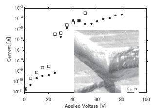
本熱電発電モジュールの性能と基板表面観察結果例
